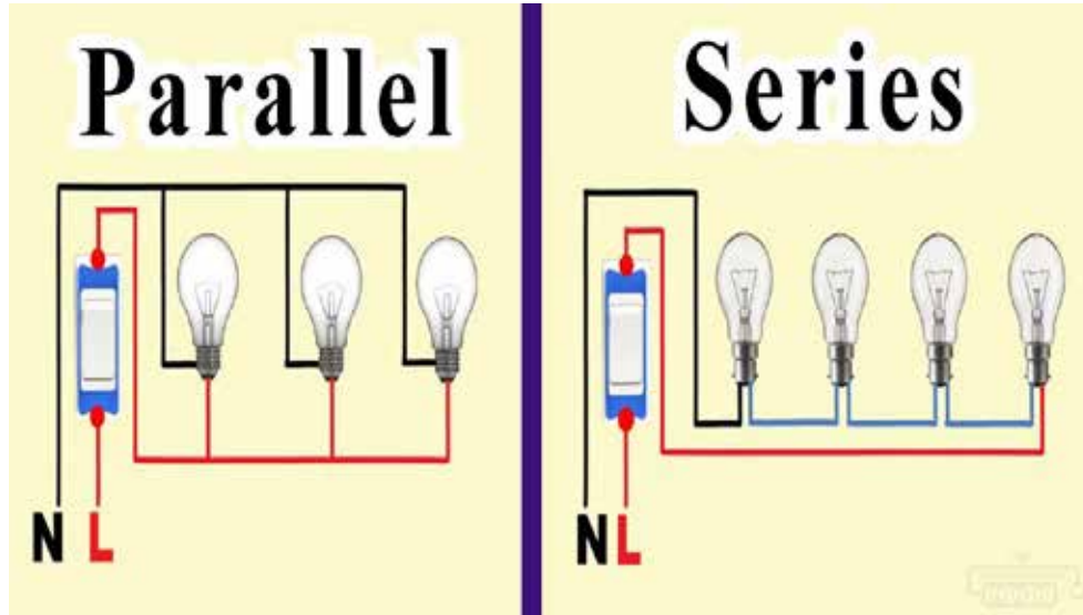
Fig 2.2.4 समानांतर और श्रृंखला वायरिंग
