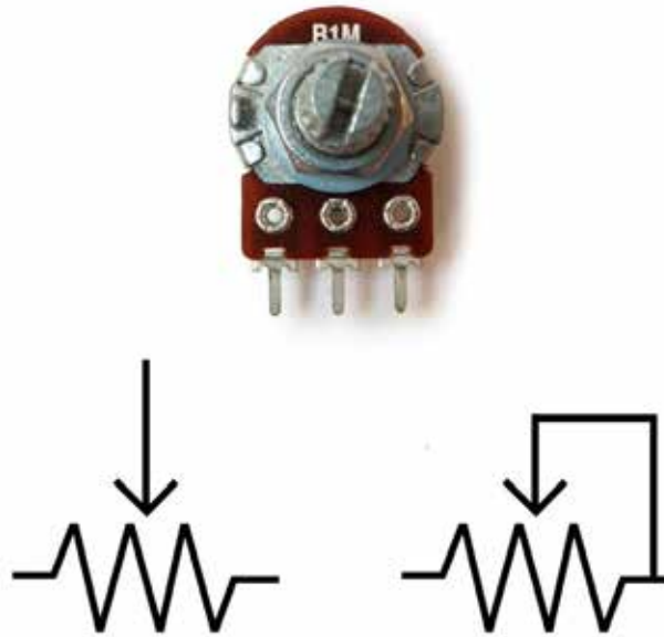
चित्र 2.3.2 (जी) विभवमापी
