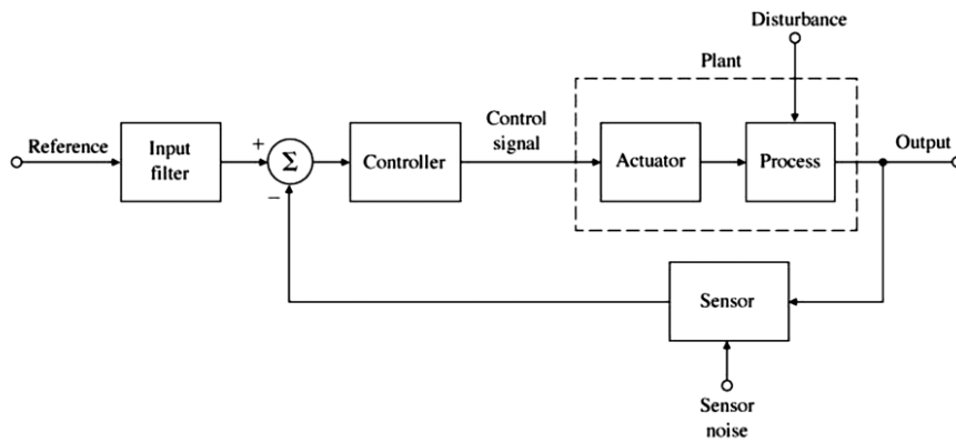
चित्र 2.2.4 (ए) ब्लॉक आरेख
