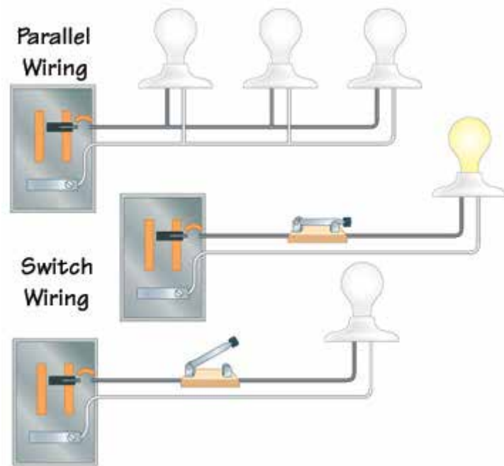
चित्र 2.2.4 समानांतर और स्विच वायरिंग
