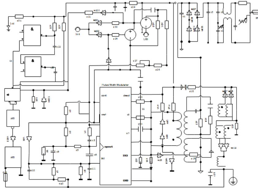
चित्र 2.2.4 (डी) वायरिंग आरेख
