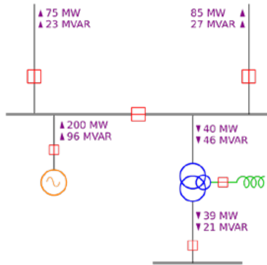
चित्र 2.2.4 (सी) रेखा आरेख
